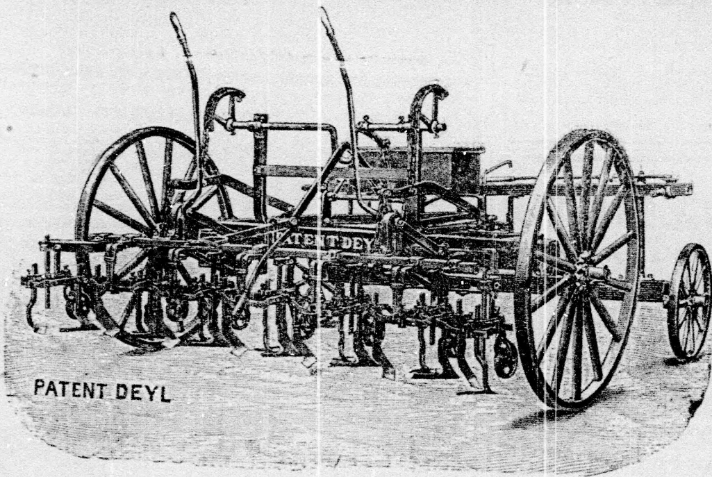
Kétfogatu kapálógépek 5-8 sorig.
