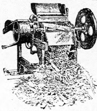
„Ohio“ kukoricaszártógép.
