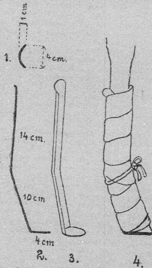
10. ábra. Csikók inróvidülésénél alkalmazandó sin és annak felkötési módja.
