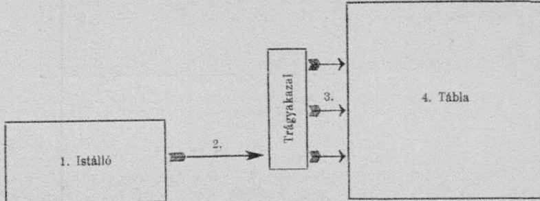
71. ábra. A tápiógyörgyei trágyakezelésnél előálló veszteségi lehetőségek bemutatása átnézeti rajzban. (Az istállótrágya levegővel érintkezik, vagyis nitrogénvesztés áll elő: 1. az istállóban, 2. a szarvasba való kihordásnál (magában a szarvasban, mivel aljára tőzeg kerül és az oldalak azonnal betapasztatnak, növényi tápanyagokban számottevő veszteség elő nem állhat), 3. a szarvasból a táblára való kihordáskor, 4. a táblán való széttergetésnél, mely után a trágyát rögtön leszántják.)
