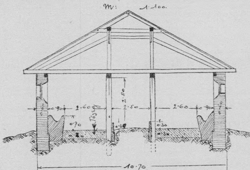
69. ábra. A tápiógyörgyei félmély istálló átmetszeti rajzban.
