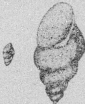
96. ábra. A kis mocsári csiga (Limnaea truncatula); baloldalt természetes nagyságban.
