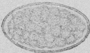
95. ábra. A nagy májmétély petéje (250-szeresen nagyítva).
