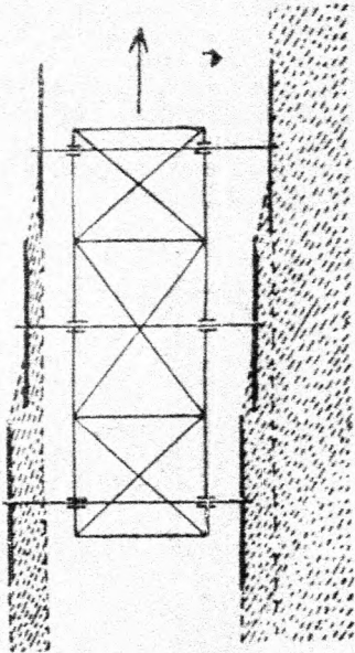
24. ábra. Két munkamenetes elrendezésti talajlazító eszköz (felülnézet).
