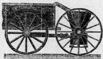
127. sz. kép. Kocsi után kapcsolt rotációs műtrágyaszóró.
