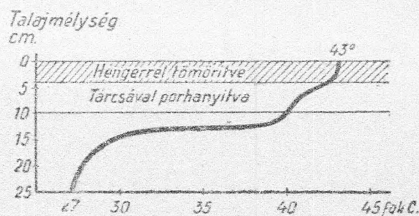
3. sz. ábra. A talajhőmérséklet változása tárcsázott és hengerrel tömörítve borsótárolóban ugyanakkor, mint az előbbiek.
