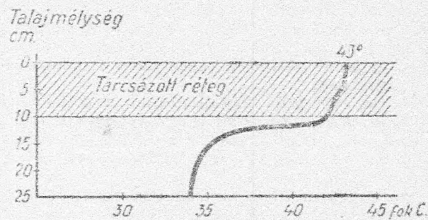
2. sz. ábra. A talajhőmérséklet változása tárcsázott (1. ábrán leírt) borsótárolóban ugyanakkor, mint az előbbiek.
