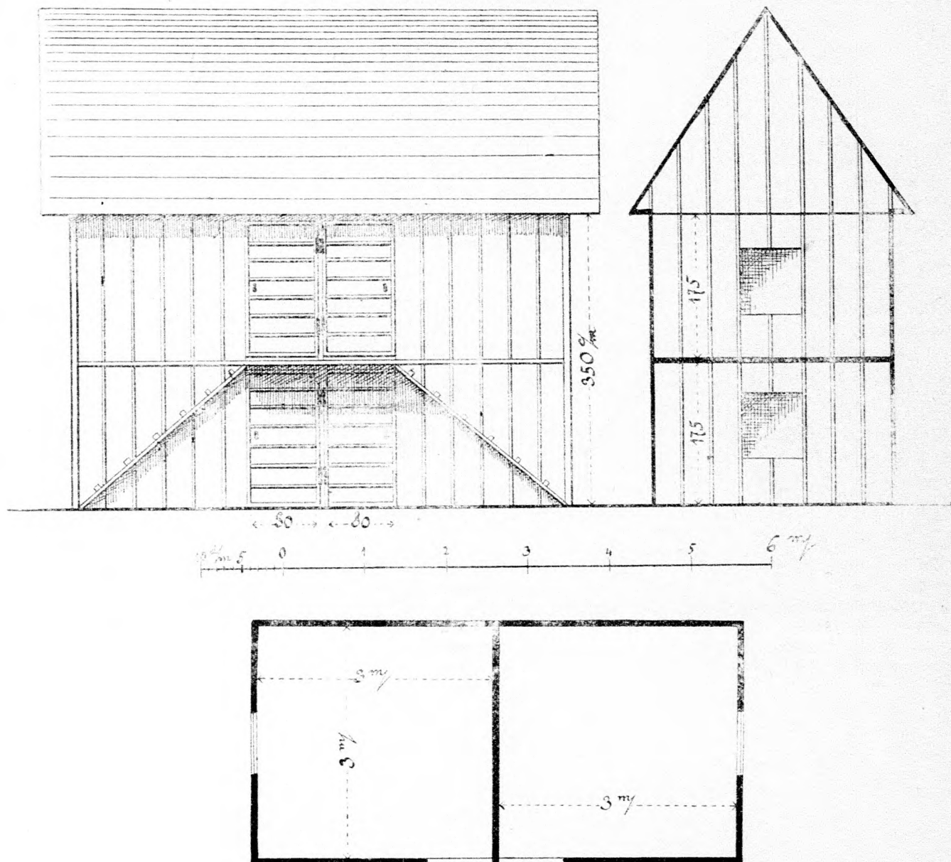
1. ábra. Baromfi-ól.
