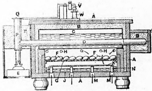
2. ábra. Kreays-féle költőgép keresztmetszete.
