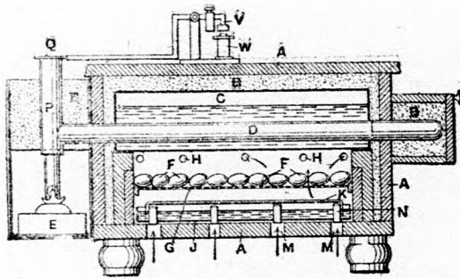
2. ábra. Kreays-féle költőgép keresztmetszete.
