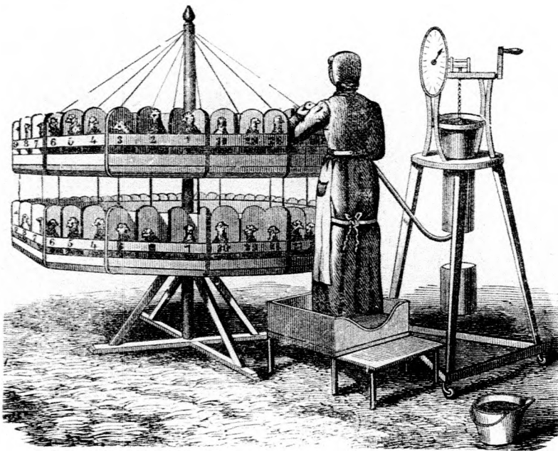
3. ábra. Két emeletes Martin Odile-féle ketrecz és tönőgép.
