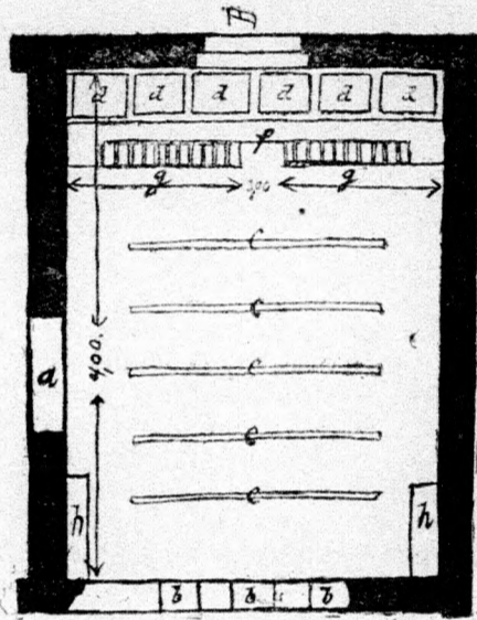
11. és 12. ábra. Viaszfehéritő berendezés.
