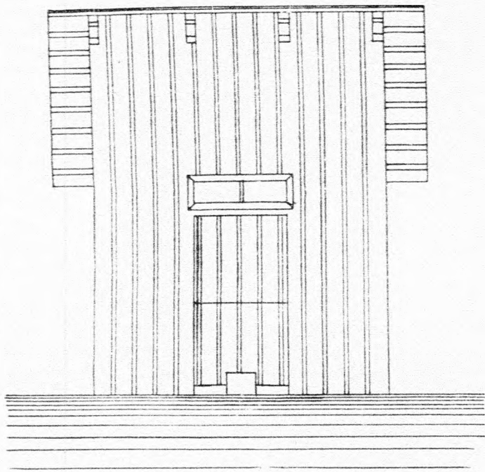
1. ábra. A tyukól homlokzata.
