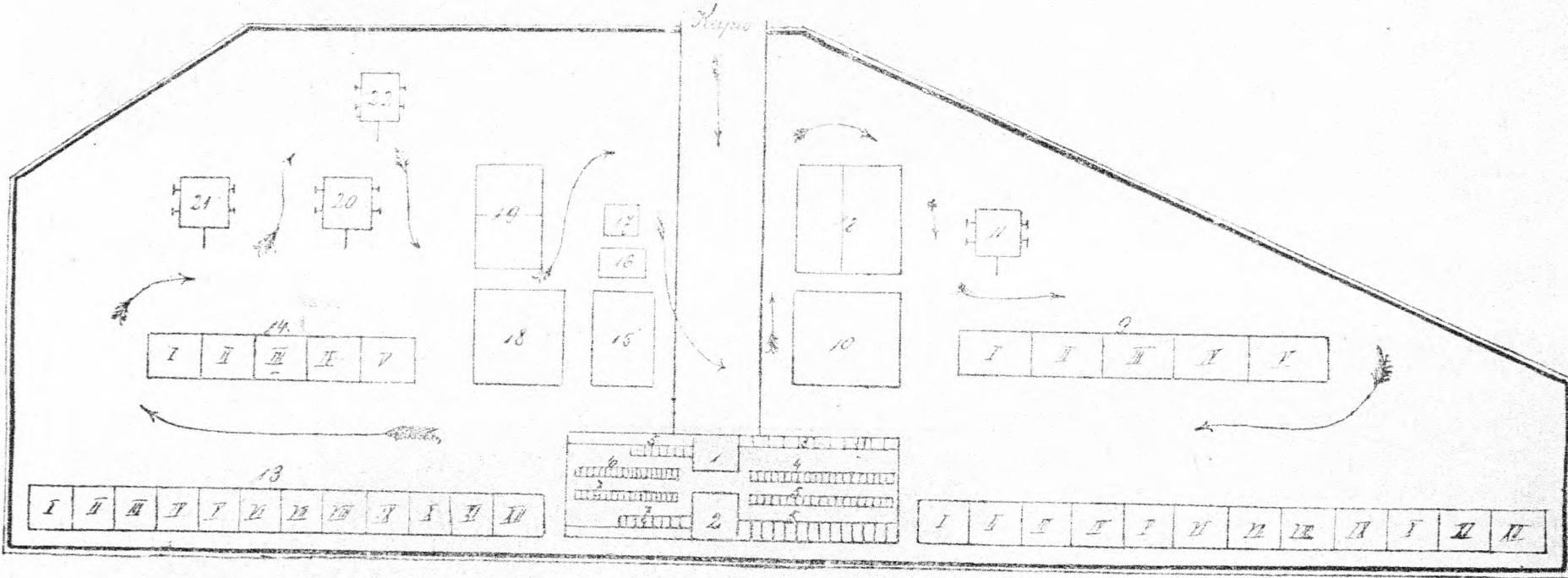
5. ábra. Baromfiállítási tervrajza.
