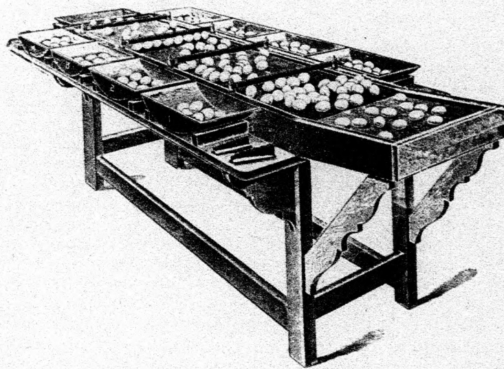
2. ábra. Tojásosztályozó gép.
