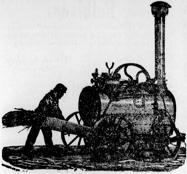
(Schlick'sches 4-pferdekräftiges Locomobil.)
