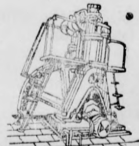
Sauggasmotor-Anlage. — Der billigste Betrieb der Gegenwart „Benz“-Rohölmotor.
