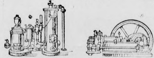
Sauggasmotor-Anlage. — Der billigste Betrieb der Gegenwart „Benz“-Rohölmotor.
