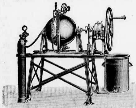
13c. sz. ábra. Ásványviz készülék.
