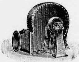
Exhaustor-Originalkonstruktion
