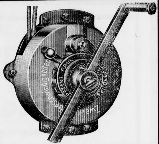
Schnellwinde für zwei Geschwindigkeiten.
