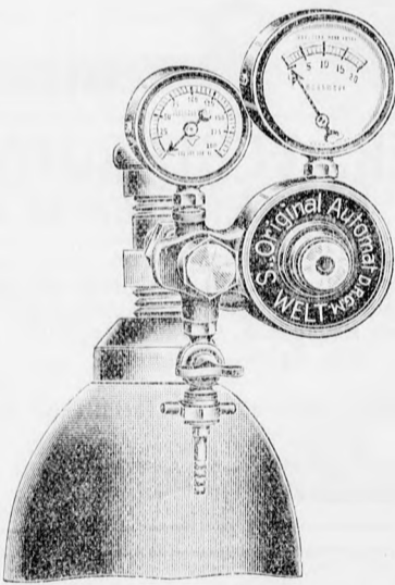
Oxigén-szelep autogén- vágáshoz.
