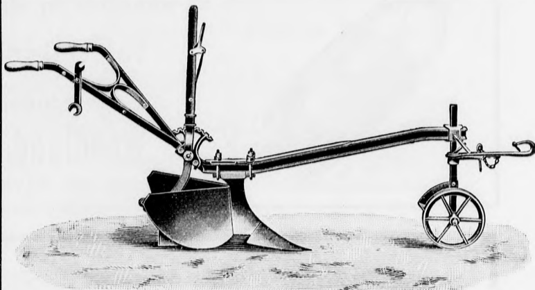
Widders neuer Häufelpflug mit Momentstellhebel. An diesen Pflug kann ein Hackkörper angeschraubt werden, der durch den gleichen Hebel in der Arbeitsbreite verstellbar ist.
