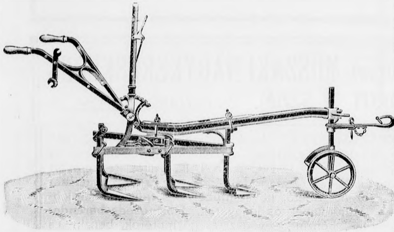
Widders Neuer Hackpflug Royal mit Momenthebelstellung. An diesen Pflug kann ein Häufelkörper angeschraubt werden, der durch Hebel in der Arbeitsbreite verstellbar ist.
