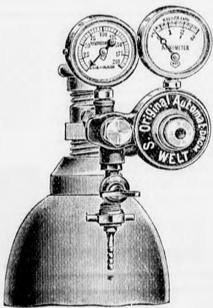
Oxigén-szelep autogén- forrasztásokhoz.
