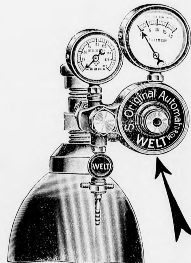
Oxigén-szelep, a nyomásmegszüntető csavar hátul. Tartalommérő központi v. központon kívüli. Mindennemű kivételben egész 40 Atm. munkanyomásig. Kiegészítés ellen védve. D. R. G. M.
