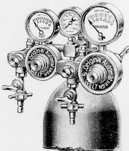
Kettős oxigén-szelep. Nyomásmegszüntető csavar elő- vagy hátsó részen. Tartalommérő központi vagy központon kívüli. Mindennemű kivételben egész 40 Atm. munkanyomásig. Kiegészítés ellen védve. D. R. G. M.
