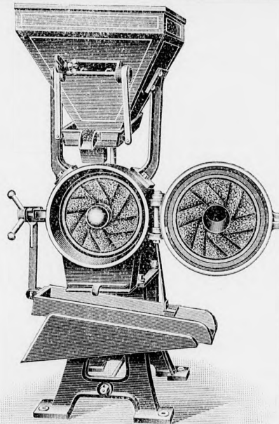
„Germania“ I. sz. tisztítás céljából nyitva.
