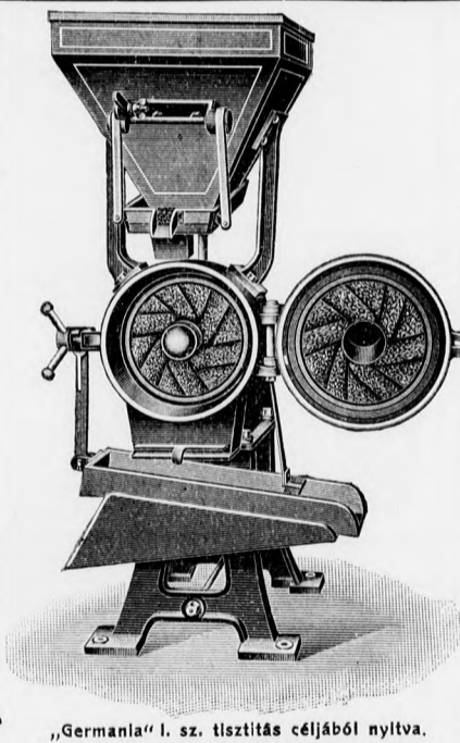
„Germania“ I. sz. tisztítás céljából nyitva.
