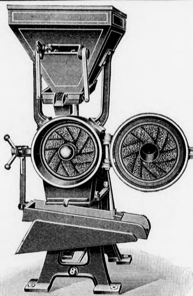
„Germania“ I. sz. tisztítás céljából nyitva.
