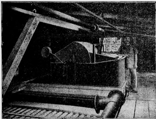
Autom. Wasserreinger System „Siegel-Simmon“ für 40.000 l. Stundenleistung
