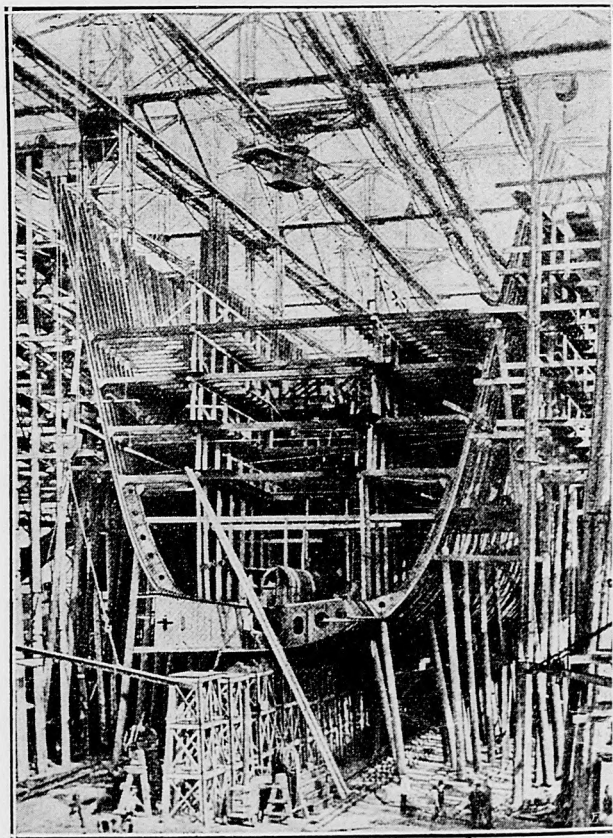
Imperator, najväčšia parolod sveta, Hamburg—amerikánskej čiary. Vystavená v hamburgskej Vulkán dielni.
