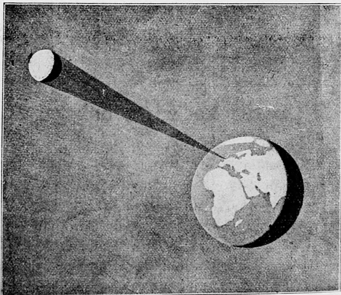
Zatmenie slnca. Malá guľa predstavuje mesiac, veľká vyobrazuje zem. Kde padá tieň mesiaca, tam nesvietí slnco a je tma na zemi.
