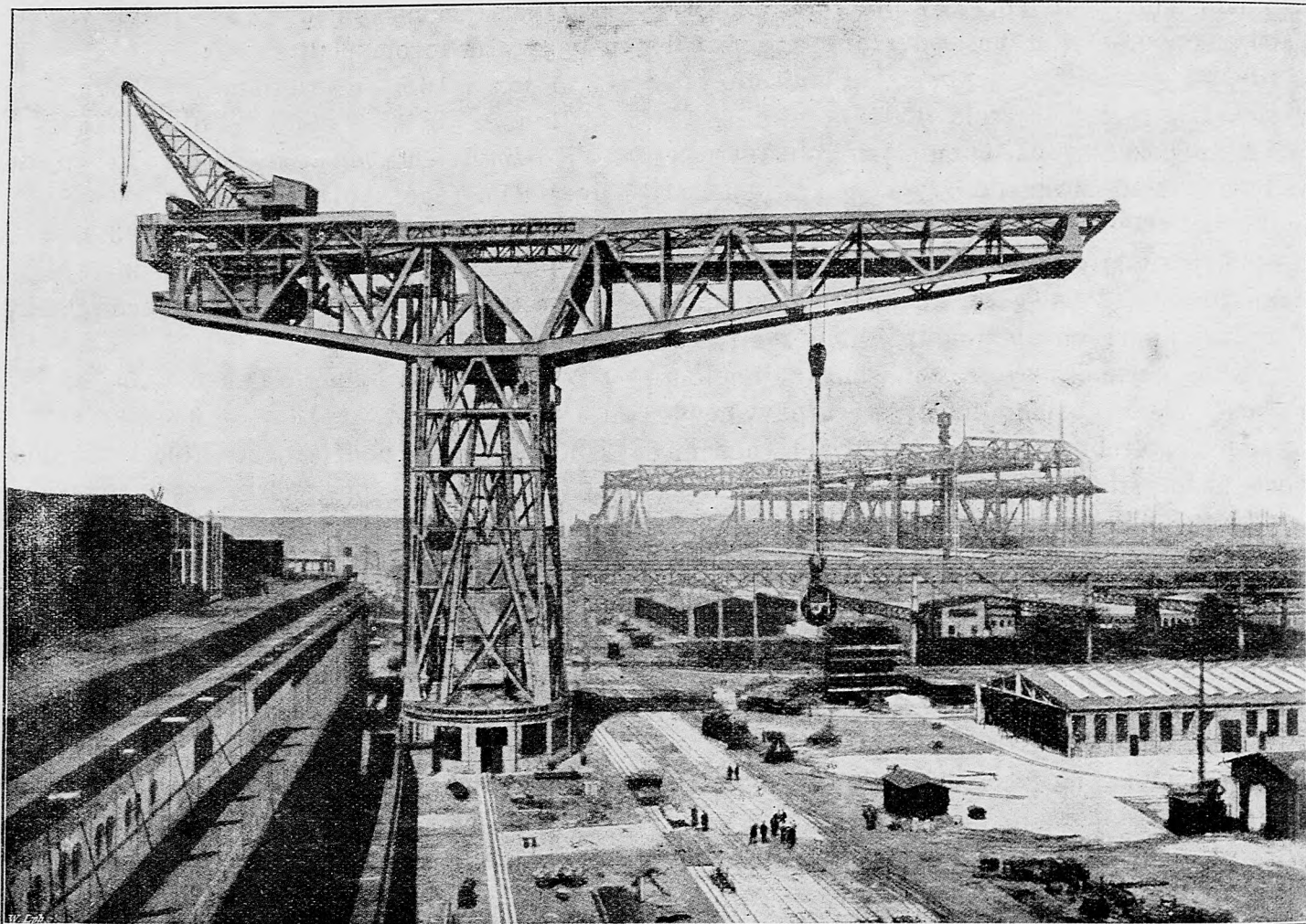
Zázrak techniky: Najväčší škrípec (elevátor) sveta v Hamburgu: vstave je sdvihnut 250 tisíc kilov. Jeho rameno je 56 metrov dlhé a 100 metrov vysoké.
