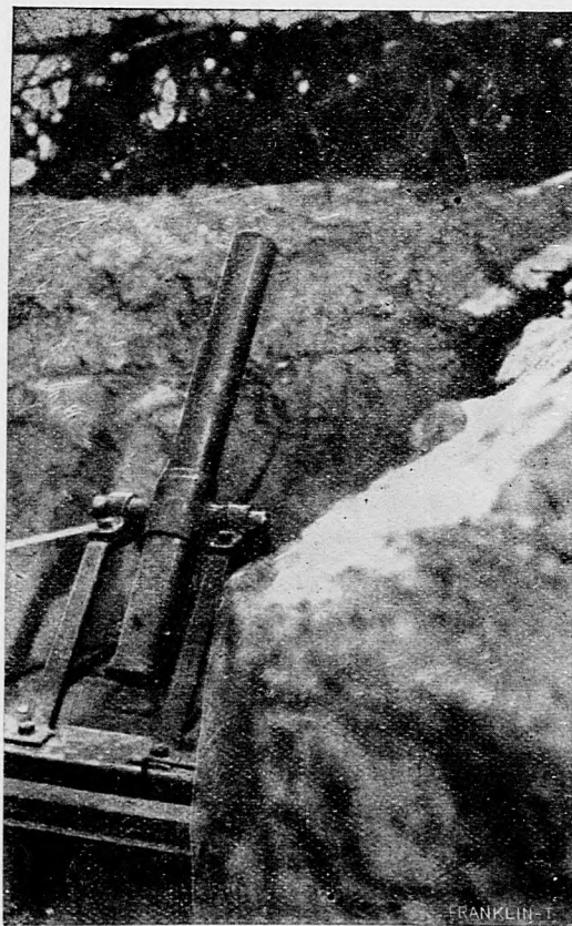
Stroj na hádzanie mín v streleckej zákope.
