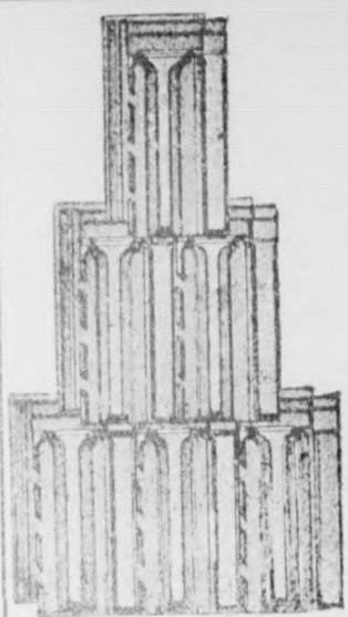
Nagykikindai gyártmány Bohn-féle szab. biztonsági átfedő-cserepek 272. sz.
