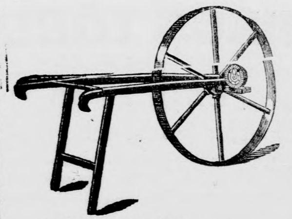
Földmérő taliga.
