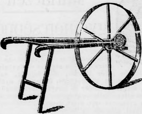
Földmérő talyiga.
