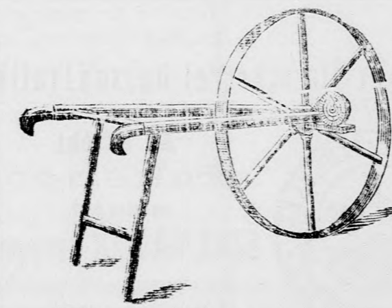
földmérő talyiga.
