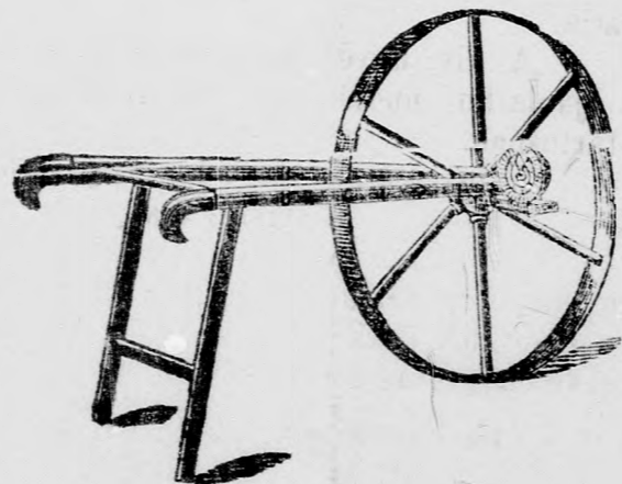
földmérő talyiga.
