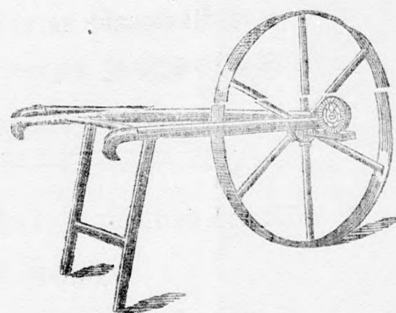
földmérő talyiga.
