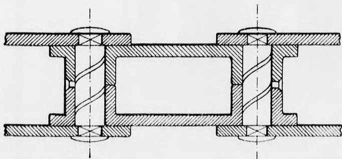
Gelenkkette mit zweitheiligen Innengliedern.
