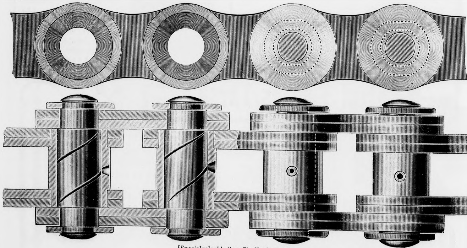
{Specialgelenkketten für Kraftantrieb.
