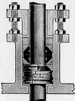
Goetze-Selbstwirkende Metall-Packung.
