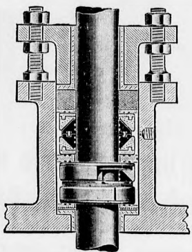
Goetze-Bewegliche, selbstwirkende Metall-Packung. D. R. P.
