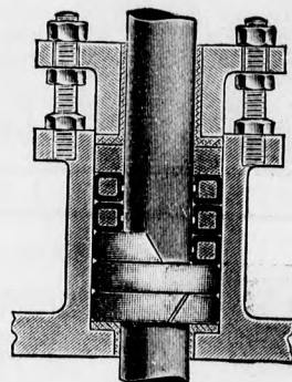
Goetze-selbstschmierende Metall-Hohring-Packung.
