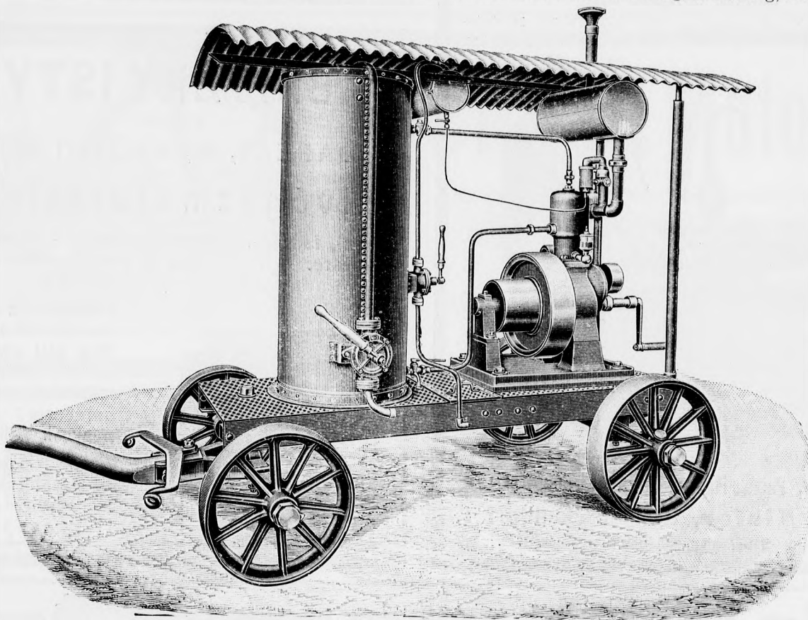
Fig. 3 „Xy“-Motor, auf einen Wagen montiert, als Benzinlokomobile.
