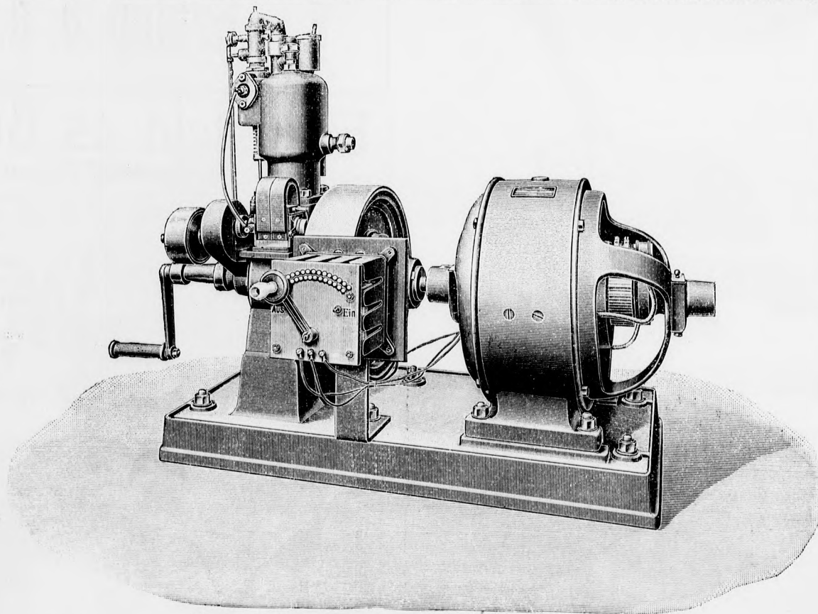
Fig. 2. „Xy“-Motor, direkt gekuppelt mit der Dynamomaschine.
