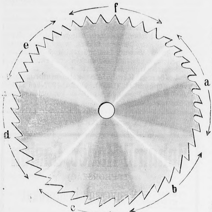
Fig. 1. Conische Metallkreissäge.
