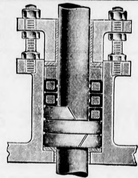
Goetze selbstschmierende Metall-Höhringpackung.
