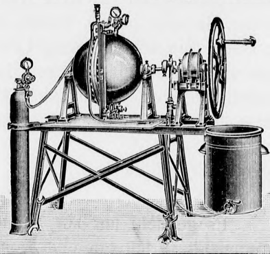
Sodawasserapparat Fig. 13c.
