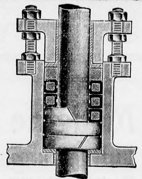
Goetze selbstschmierende Metall-Hohlringpackung.
