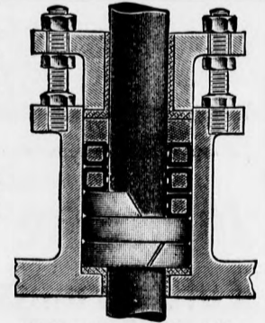
Goetze selbstschmierende Metall-Hohlringpackung.
