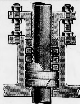
Goetze selbstschmierende Metall-Hohlringpackung.
