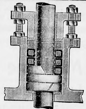
Goetze selbstschmierende Metall-Hohringpackung.
