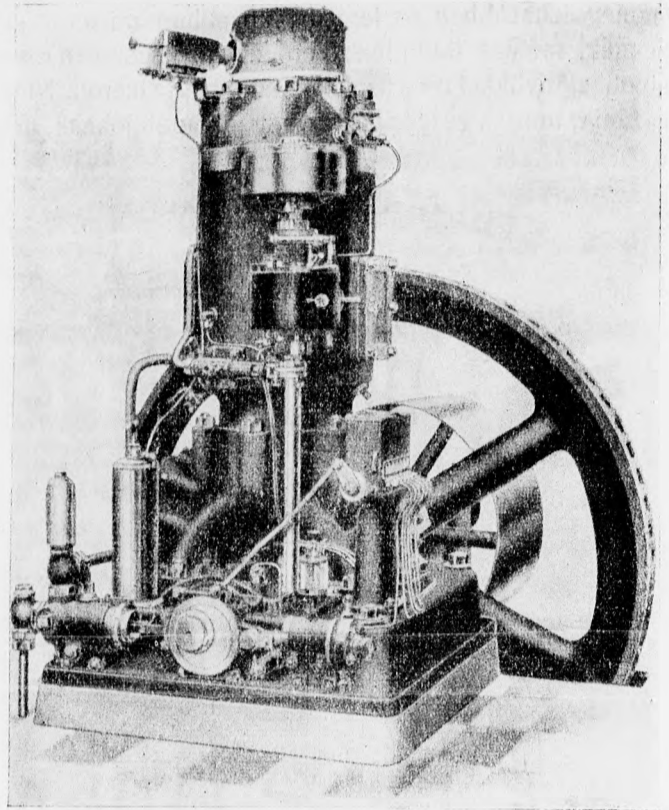
4. ábra. Egy-cylinderes Swiderski-nyersolajmotor 18—60 HP.
