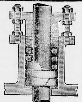
Goetze selbstschmierende Metall-Hohringpackung.
