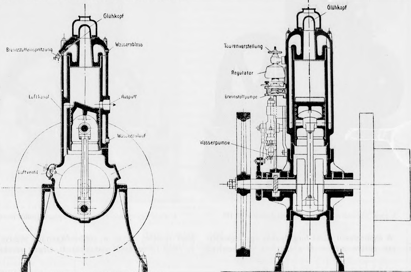
1. és 2. ábra. Swiderski-nyersolajmótor keresztmetszetei.
