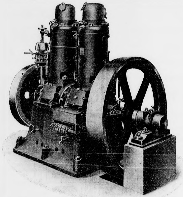
3. ábra. 2-cylinderes Swiderski-nyersolajmotor 30 HP.
