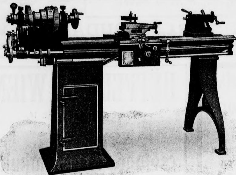
Präzisions-Zug- und Leitspindel-Drehbank „Universal.“
