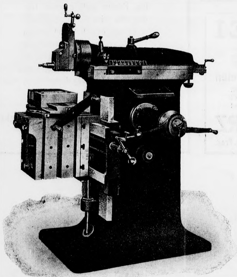
Shapingmaschine, 430 mm. Stößelhub.
