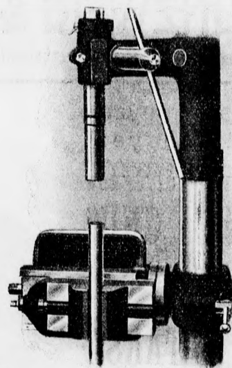
Bohrtisch mit Schraubstock, drehbar, anerkannt praktisch.
