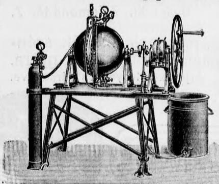
Sodawasserapparat Fig. 13c.
