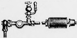
Rohrreiner wie im Gebrauch für Pressluft und Dampf.
