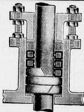
Goetze selbstschmierende Metall-Hohringpackung.
