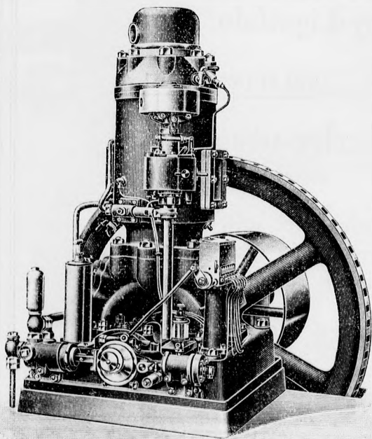
35 HP 2 cylinderes kivitel.
