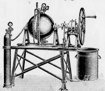
Sodawasserapparat Fig. 13c.
