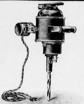
Elektrische Hand- und Tisch-Bohr- maschinen mit 1, 2 und 3 Ge- schwindigkeiten für Gleich- und Wechselstrom.
