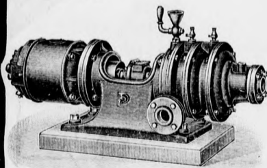
Turbinen-Pumpe, ein- u. mehrstufig, direkt gekuppelt mit angeflanschem Elektromotor.
