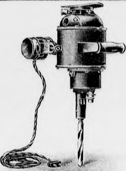
Elektrische Hand- und Tisch-Bohrmaschinen mit 1, 2 und 3 Geschwindigkeiten für Gleich- und Wechselstrom.
