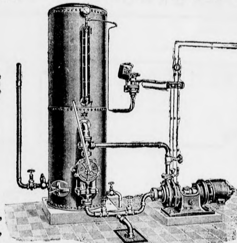
Hauswasserversorger „Hydrophor“ D. R.-G.-M. Elektrisch-automatisch, für Hand- u. Motorbetrieb, ca. 2500 Anlagen geliefert.
