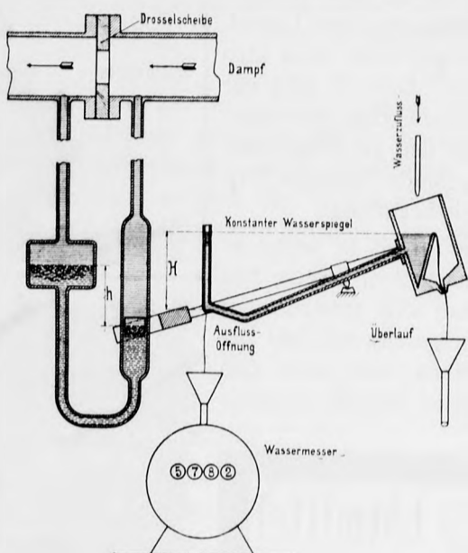
Abb. 2. Dampfmesser „Badias“.
